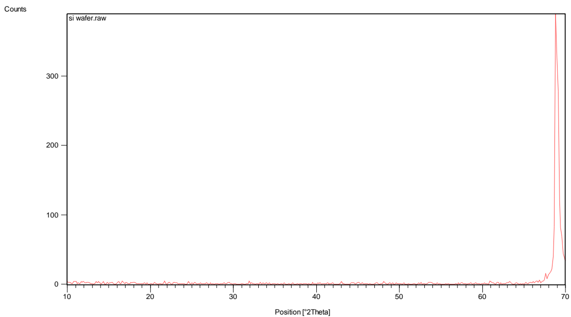
طیف اولیه نمونه ویفر سیلیکون تک کریستال مربوط به دکتر رسولی بعد از تنظیمات در تاریخ ۹۷/۱۱/۸
