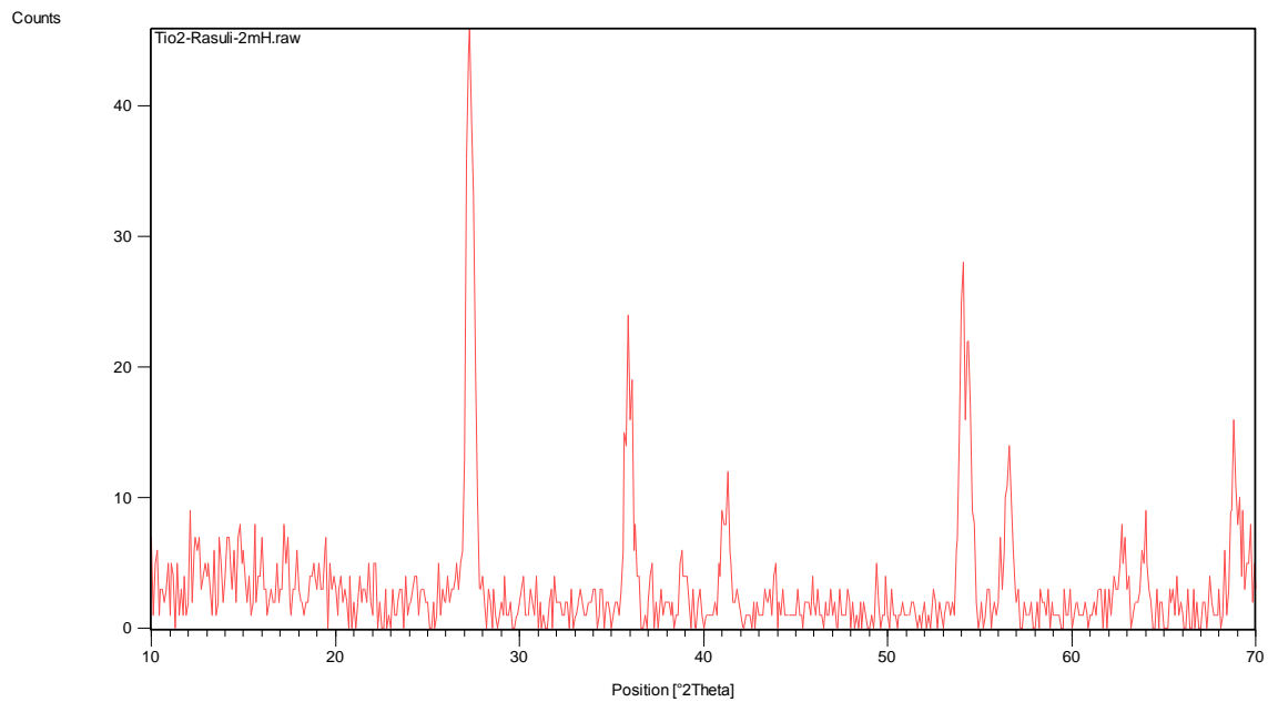
طیف اولیه نمونه آزمایشگاهی نانوذرات TiO_2 مربوط به دکتر رسولی بعد از تنظیمات در تاریخ ۹۷/۱۱/۸
