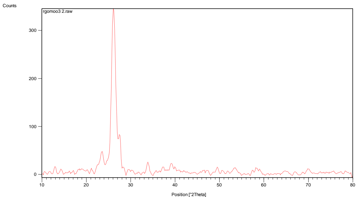
طیف اولیه نمونه آزمایشگاهی نانوذرات \text{RGOMoO}_3 مربوط به دکتر رسولی بعد از تنظیمات در تاریخ ۹۷/۱۱/۱۰
