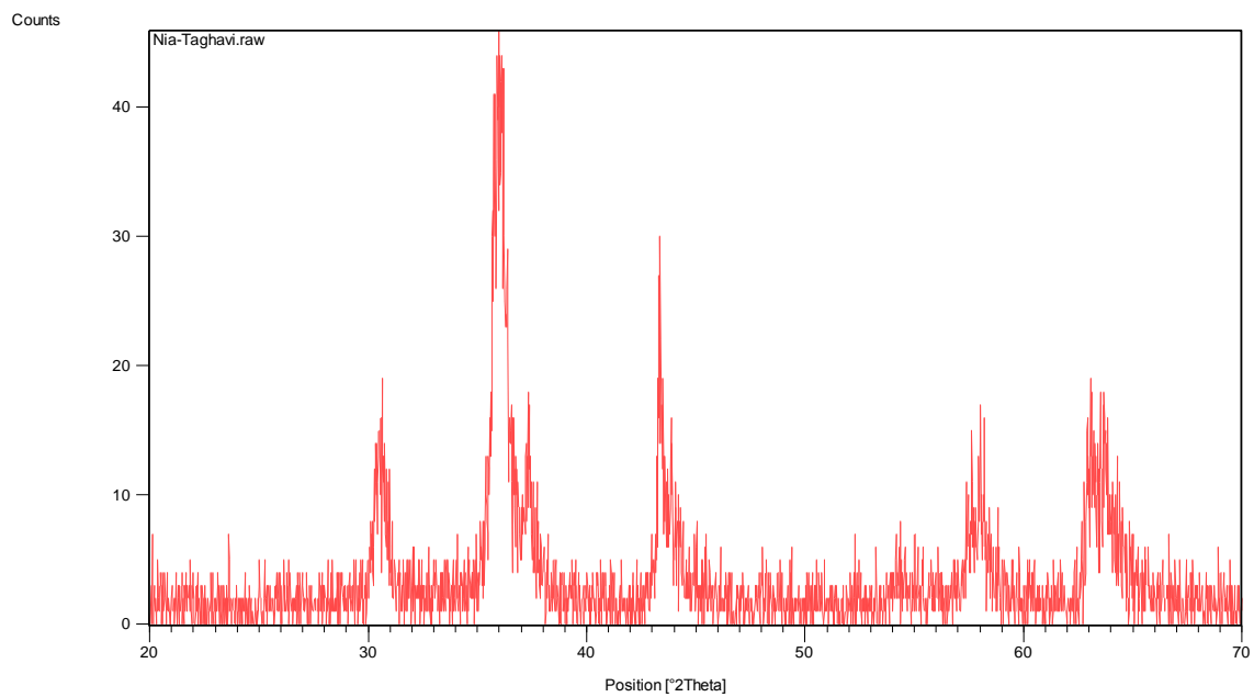
طیف اولیه نمونه آزمایشگاهی نانوذرات \text{TiO}_2 مربوط به دکتر رضانی قبل از تنظیمات در تاریخ ۹۷/۱۱/۸
