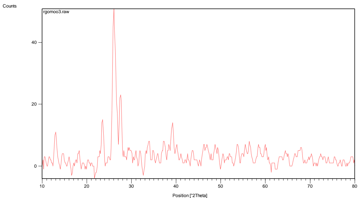
طیف اولیه نمونه آزمایشگاهی نانوذرات \text{RGOMoO}_3 مربوط به دکتر رسولی قبل از تنظیمات در تاریخ ۹۷/۱۱/۸ و ۹۷/۱۱/۱۰
