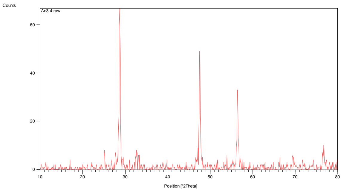
طیف اولیه نمونه خاک معدن انگوران مربوط به دکتر نباتیان بعد از تنظیمات در تاریخ ۹۷/۱۱/۸
