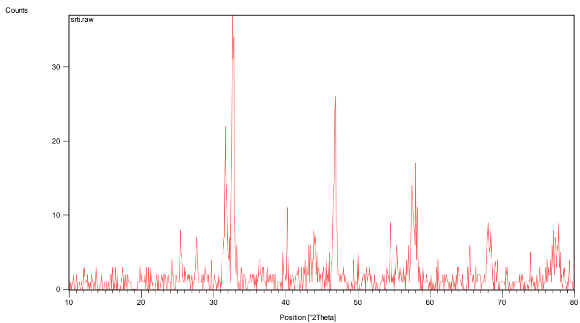
طیف اولیه نمونه آزمایشگاهی نانوذرات SrTi مربوط به دکتر رضانی قبل از تنظیمات در تاریخ ۹۷/۱۱/۸
