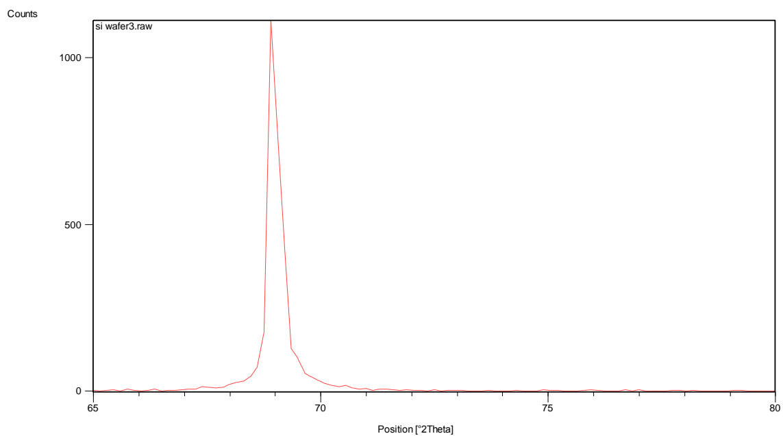
طیف اولیه زوم شده نمونه ویفر سیلیکون تک کریستال مربوط به دکتر رسولی بعد از تنظیمات در تاریخ ۹۷/۱۱/۸
