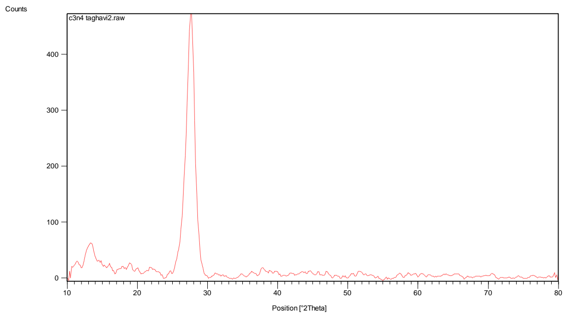
طیف اولیه نمونه آزمایشگاهی C_3N_4 مربوط به دکتر رضانی بعد از تنظیمات در تاریخ ۹۷/۱۱/۱۰ توان مورد استفاده دستگاه ۸۷۵ وات
